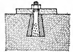
Rag Bolt.
