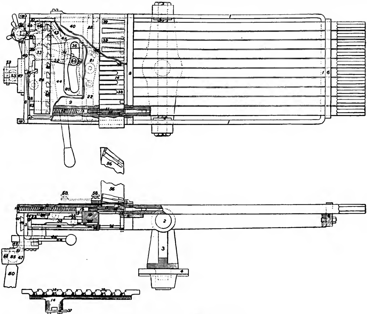
FIG. 5.—Nordenfeldt Machine-Gun.
